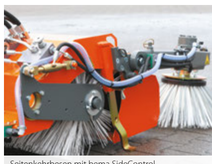
Seitenkehrbesen mit bema SideControl und Wassersprüheinrichtung
